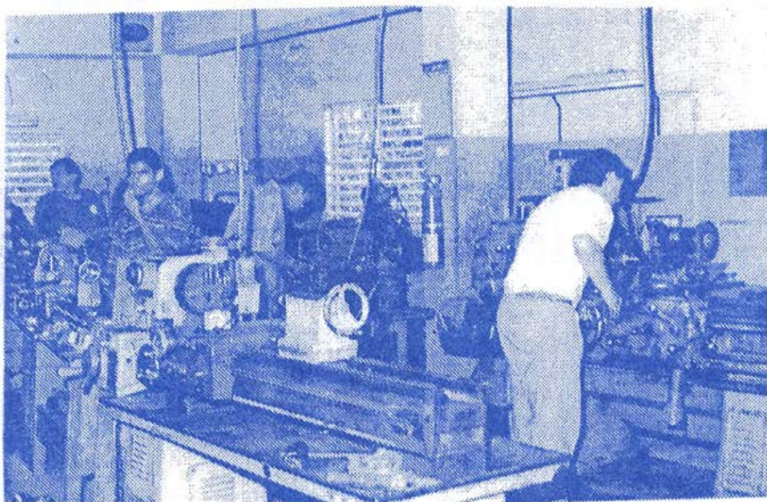
Se observa el taller del Sr. Julio Brache, beneficiario de préstamo. Este taller cuenta con 14 empleados fijos y se dedica a la rectificación de cilindros de motores para motocicletas y vehículos. Es el único que existe en esta Provincia.
